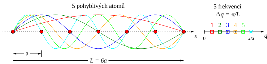
Obr. 6.1: Řetízek sedmi atomů s fixními okrajovými podmínkami.
