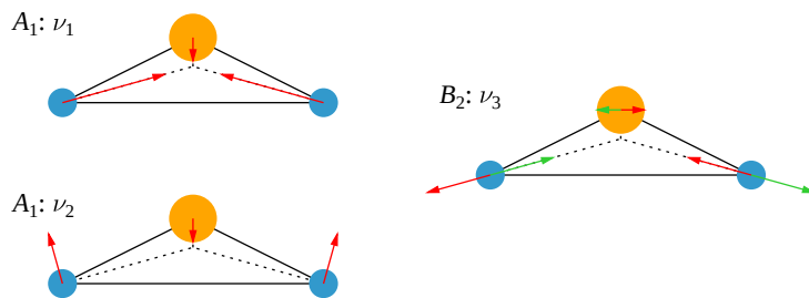
Obr. 2.4: Vibrační módy molekuly vody a jejich symetrie popsaná NIR.
