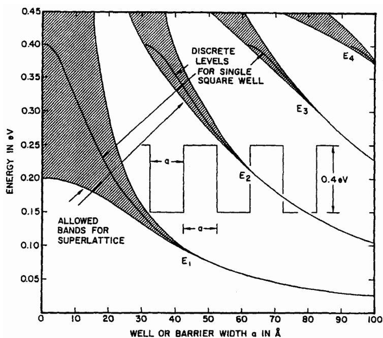
Obr. 12.7: Závislost polohy a šířky elektronových energetických podpásů supermřížky na šířce jámy (šířka bariéry je stejná jako šířka jámy). Převzato z [23].
