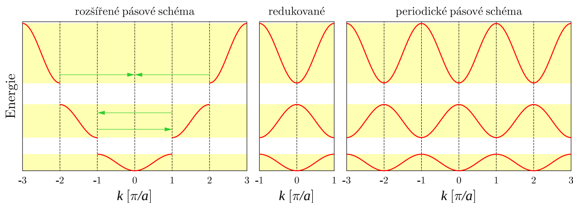
Obr. 10.1: Energetické pásy 1D řetízku zakreslené zleva v rozšířeném, redukovaném a periodickém pásové schématu. Zelené šipky ukazují vektor \vec{G} odpovídající šířce BZ, o který se provádí posun energetických závislostí.
