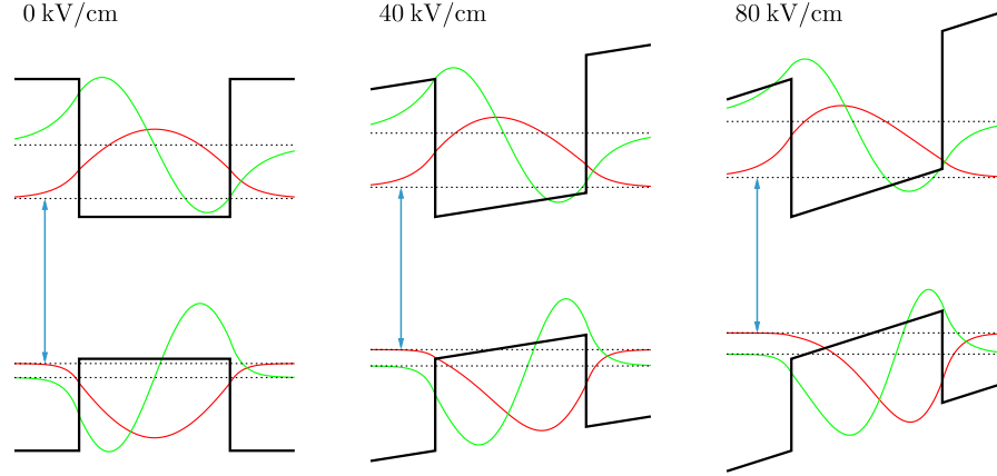
Obr. 12.6: Černá čára představuje profil vodivostního a valenčního pásu pro kvantovou jámu GaAs šířky 10 nm obklopenou Ga 0.7 Al 0.3 As. Pásky jsou nakloněny vyznačeným elektrickým polem. V tomto potenciálu jsou spočítány první dvě hladiny pro elektrony a těžké díry podle (12.20). Modrou šipkou je zakreslena vzdálenost základní elektronové a děrové hladiny.
