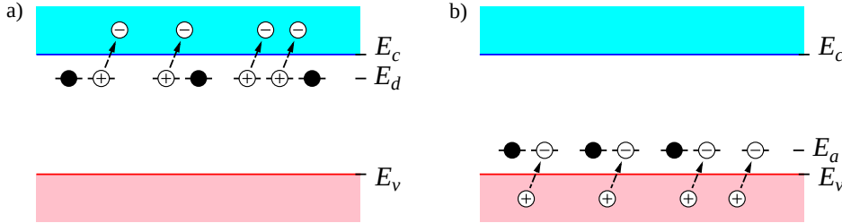
Obr. 9.13: Ionizace příměsí v polovodiči: a) n-typ s donory, b) p-typ s akceptory. Energie E_v a E_c označují hranu valenčního, resp. vodivostního pásu.
