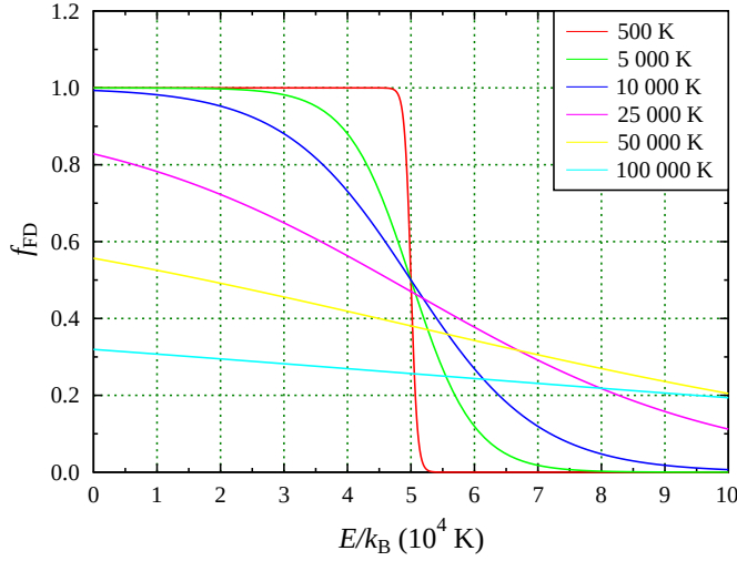
Obr. 7.2: Fermiho-Diracova distribuční funkce (7.5) pro různé teploty s typickou Fermiho teplotou pro kovy T_F = E_F/k_B = 5 \times 10^4 K.
