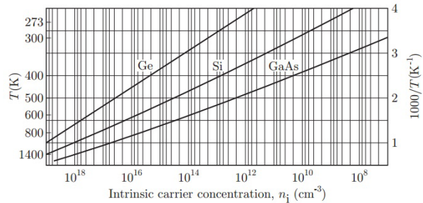
Obr. 9.11: Teplotní závislost koncentrace elektronů pro tři různé polovodiče [21].
