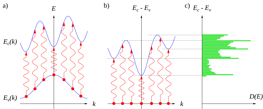
Obr. 11.4: Optická mezipásová absorpce: a) Obecné pásové schéma, červeně jsou vyznačeny fotoexcitované mezipásové přechody; b) zobrazení energie optického přechodu v různých místech BZ; c) sdružená hustota stavů jako histogram z b).
