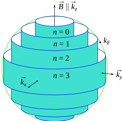
Obr. 10.15: Znáznornění 3D Landauových energetických hladin v k -prostoru. Index n značí číslo hladiny podle (10.35), zeleně je zakreslena poloha Fermiho meze pro případ bez magnetického pole.
