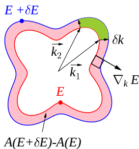
Obr. 10.13: Geometrická interpretace parametrů použitých v textu. Rovina nákresu je kolmá na magnetické pole. Červeně je zakreslena orbita s energií E a modře orbita s energií E + \delta E . Růžová plocha označuje rozdílovou plochu mezi orbitami. Zelená část představuje integrál mezi body \vec{k}_1 a \vec{k}_2 podle vztahu (10.24) a je úměrný rozdílu času (t_2 - t_1) .
