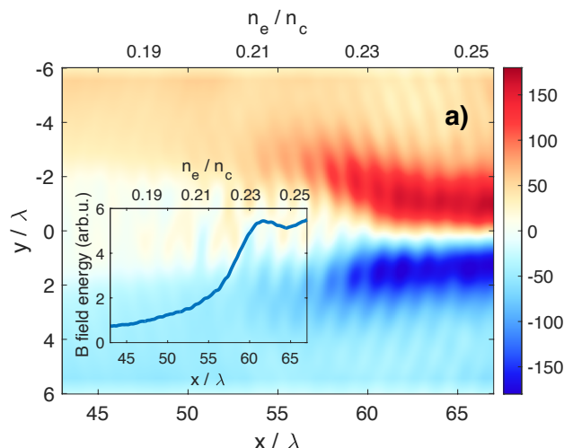
Obrázek 1: Silné magnetické pole vznikající při interakci svazku laseru PALS s plazmatem v oblasti kritické hustoty – výsledek z 3D PIC simulace.
